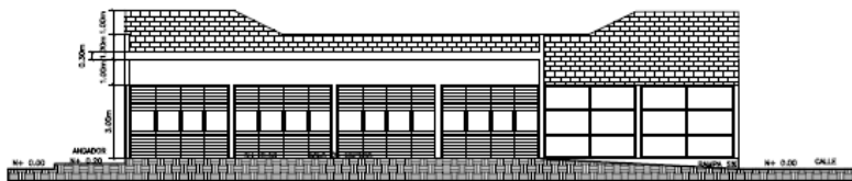
SECCION A-A''
